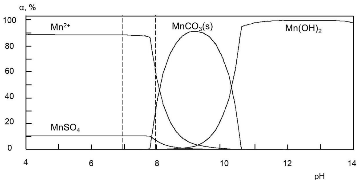
Рисунок 5.5 – Графік залежності форм знаходження \text{Mn}^{2+} (у відсотках) у воді від величини рН середовища (умовно чиста територія, склад води гідрокарбонатний магнієво-кальцієвий), штрих пунктиром позначено межі рН
