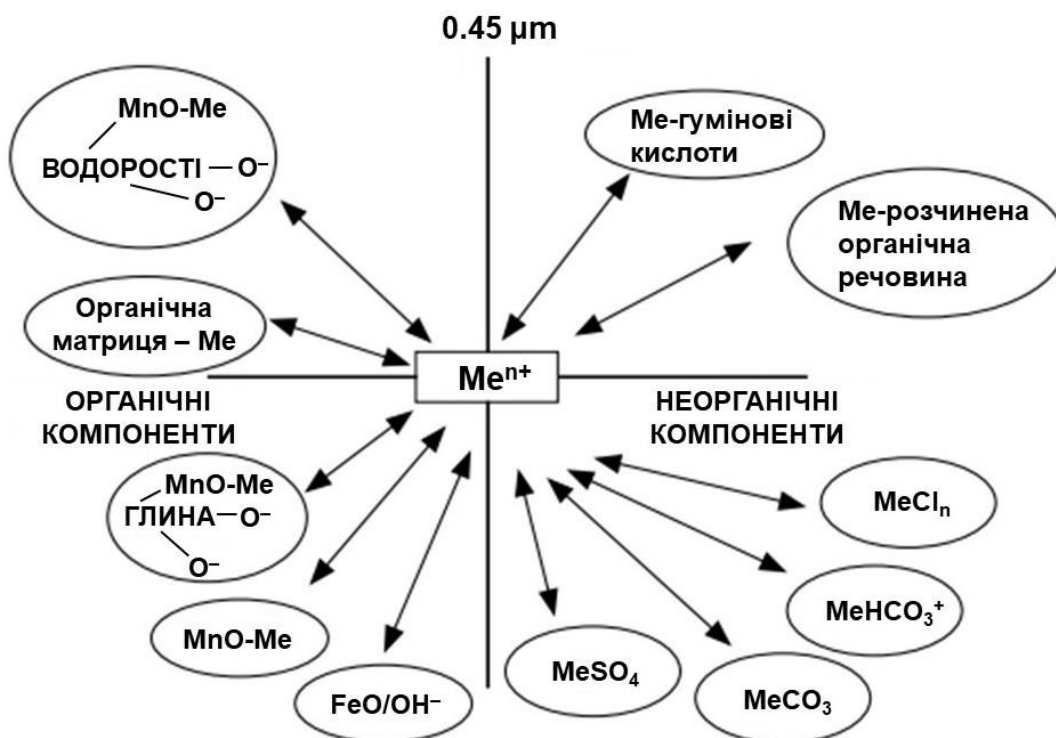
Рисунок 2.2 – Схематичне представлення рівноваги між іонами металів та лігандами органічної та неорганічної природи у водному середовищі: розчинений та нерозчинений стан компонентів відносно фільтру 0.45 \mu\text{m} (Bjerregaard & Andersen, 2014)
