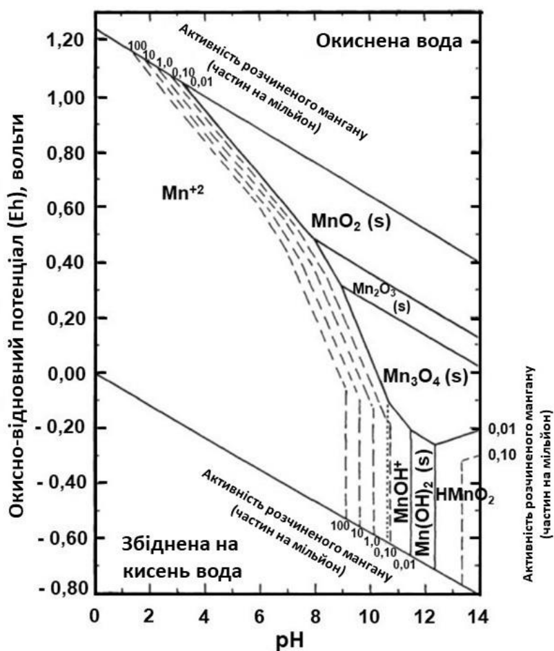
Рисунок 5.2 – Діаграма Eh-pH, що описує стабільність твердої «(s)» і водної фаз мангану як функцію окисно-відновного потенціалу і рН, за стандартної температури (25°C) і тиску (1 атмосфера). У твердих стабілоях манган випадає в осад з утворенням нерозчинної сполуки. Поля стабільності твердих речовин (суцільні лінії) являють собою межі за концентрацій 0,01 ppm (часток на мільйон) розчиненого мангану ( \text{мкг/дм}^3 ). Пунктирні лінії представляють межі поля стабільності, коли концентрації розчиненого Mn^{+2} становлять 0,10; 1,0; 10 і 100 ppm (Нem, 1985)
